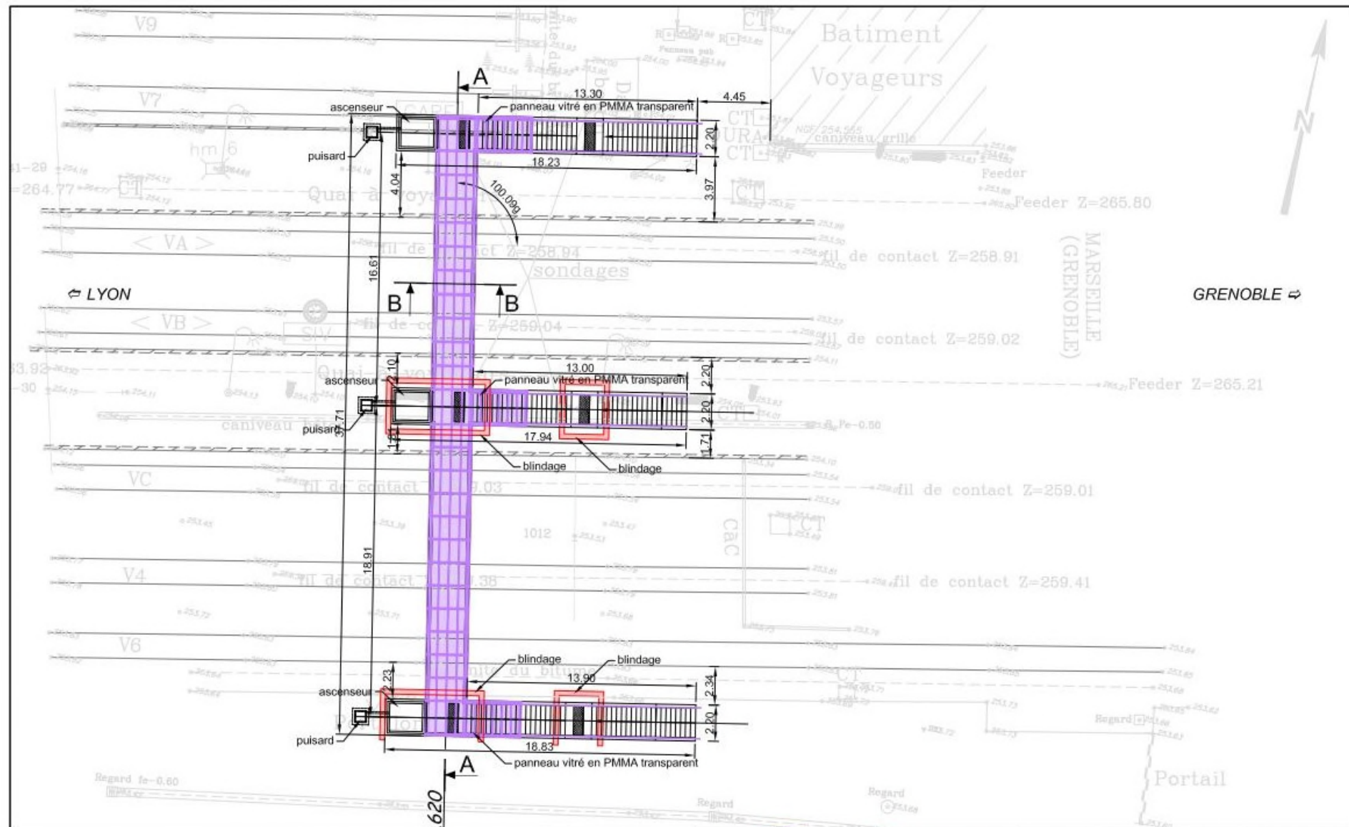
VUE EN PLAN éch. 1/200
